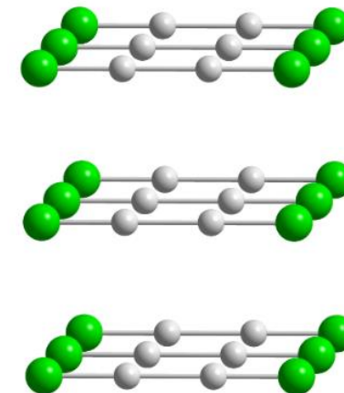
molekulový \text{Hg}_2\text{Cl}_2
