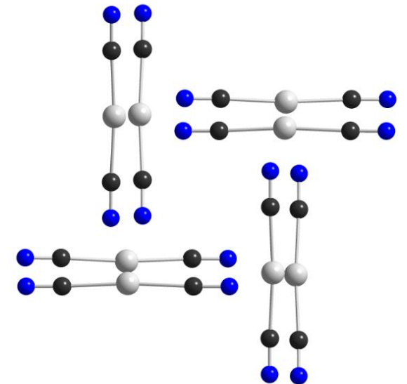
Molekulová štruktúra \text{Hg}(\text{CN})_2 80
