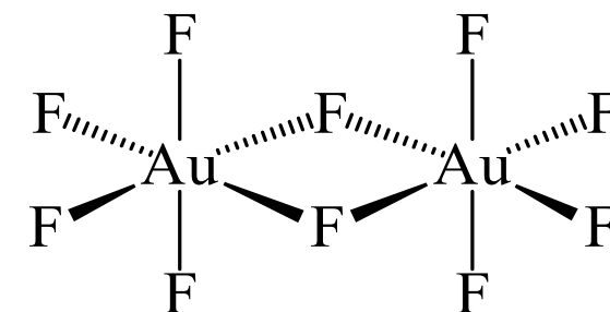
Au 2 F 10
