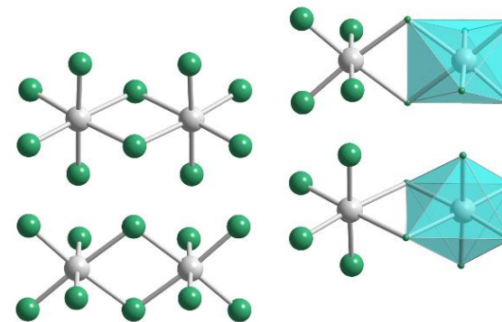
dimérny \text{AuF}_5
