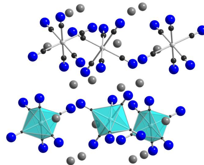
iónová štruktúra \text{K}_3[\text{Cr}(\text{CN})_6]
