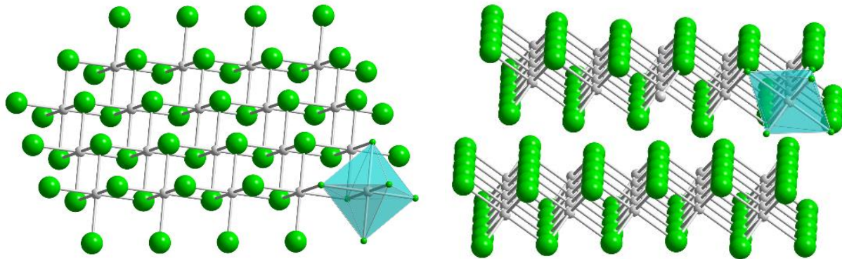
Vrstevnatá polymérna štruktúra \text{FeCl}_2
