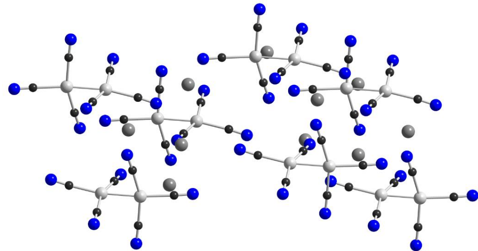
Molekulová štruktúra \text{K}_4[\text{Ni}_2(\text{CN})_6]
