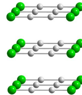
\text{Hg}_2\text{Cl}_2
