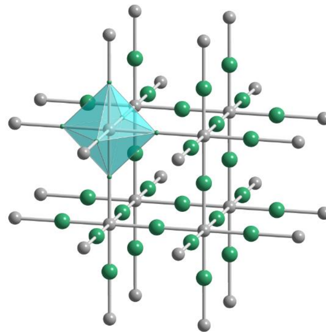
Niggliho vzorec \{\text{ScF}_{6/2}\}
