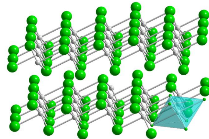
\text{CuCl}_2
