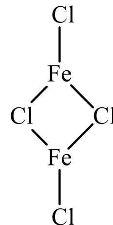
dimérna štruktúra plynného (\text{FeCl}_2)_2
