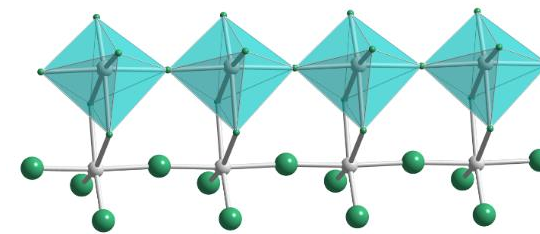
Reťazcová polymérna štruktúra \text{CrF}_4
