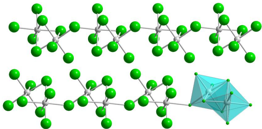
Reťazcová polymérna štruktúra \text{ReCl}_4
