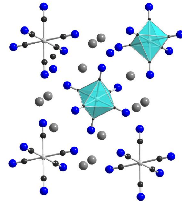
Kryštálová štruktúra iónového K 3 [Fe(CN) 6 ]
