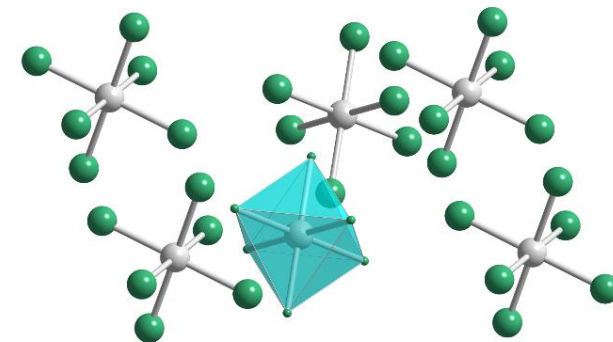
oktaédrické molekuly PtF 6
