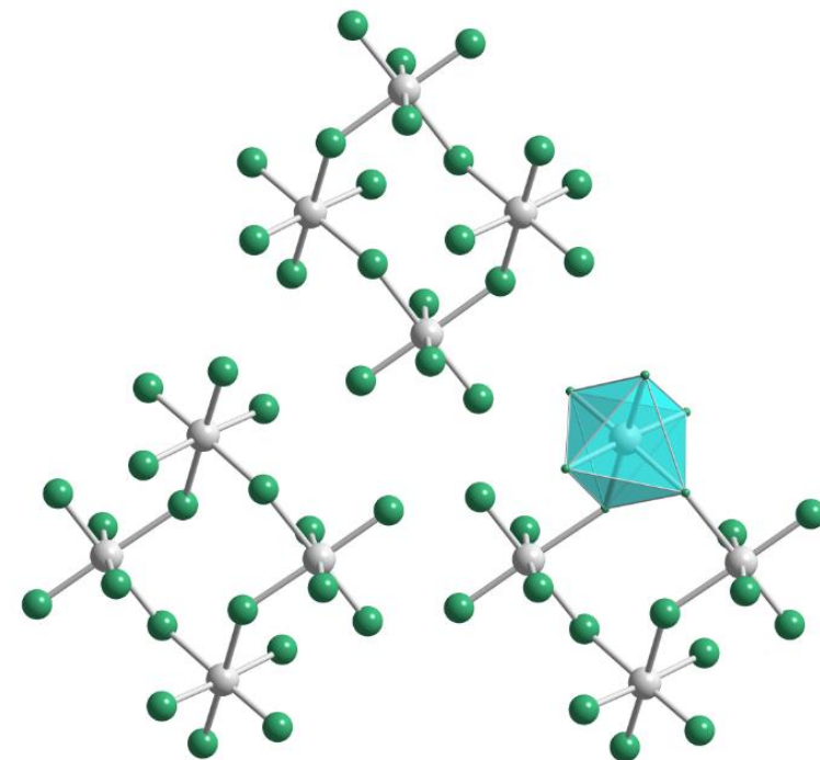
tetramérne molekuly (PtF 5 ) 4 .
