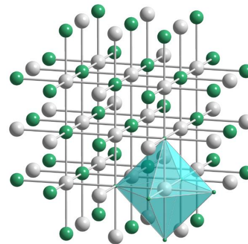
Iónová struktúra AgF
